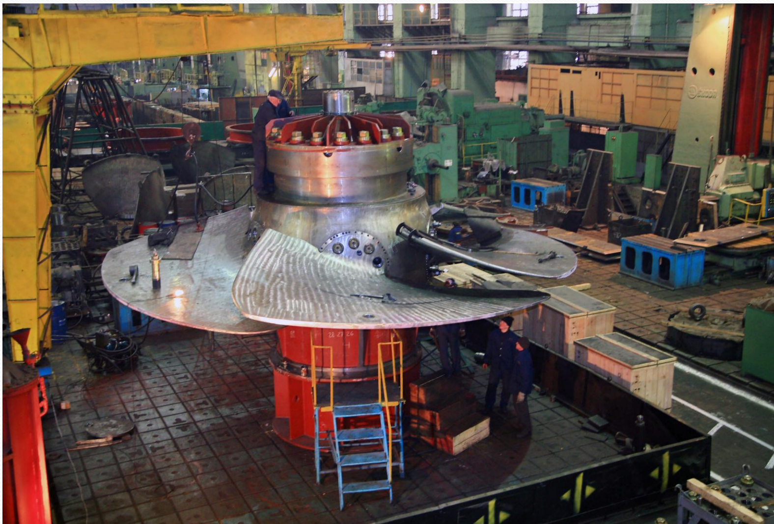
Поворотно-лопастное рабочее колесо для гидротурбины Новосибирской ГЭС
