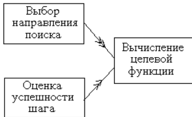
Рис. 12. IDEF4-диаграмма клиентов
