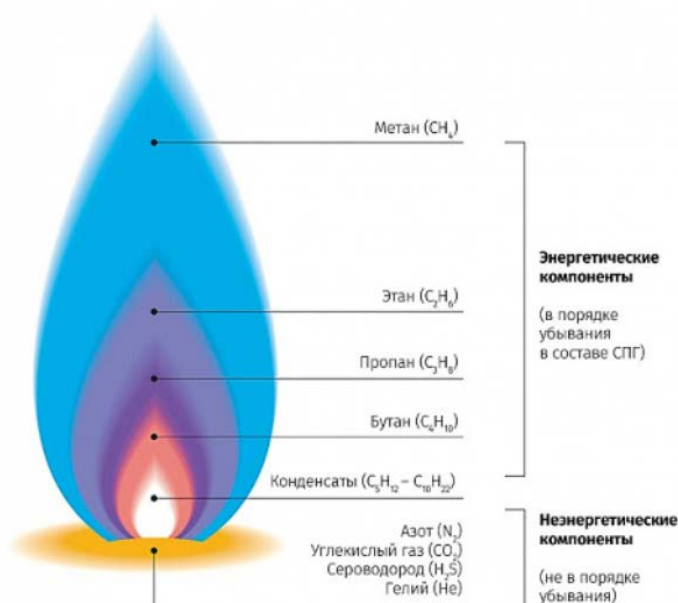
Рисунок 1.2 – Компоненты газа.
