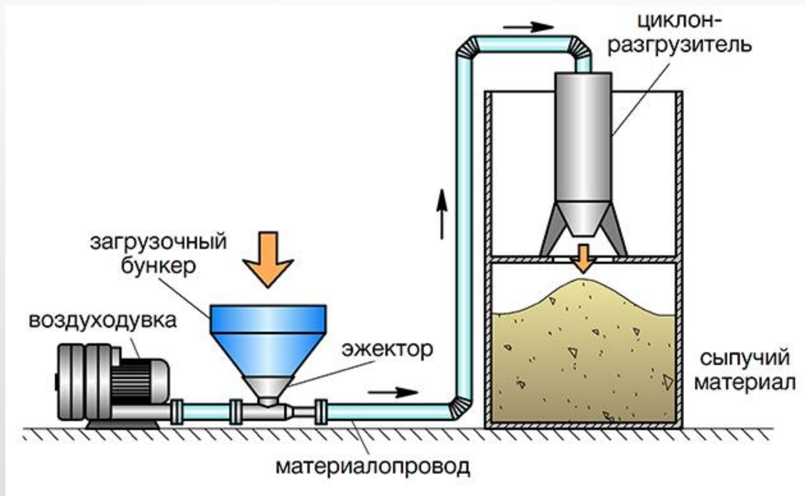
Рисунок 1. – Пневмотранспорт
