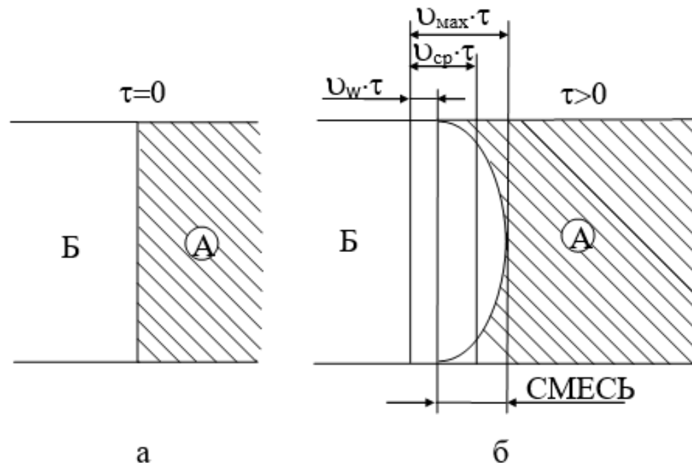
Рисунок 1.2- Механизм смесеобразования при турбулентном режиме
