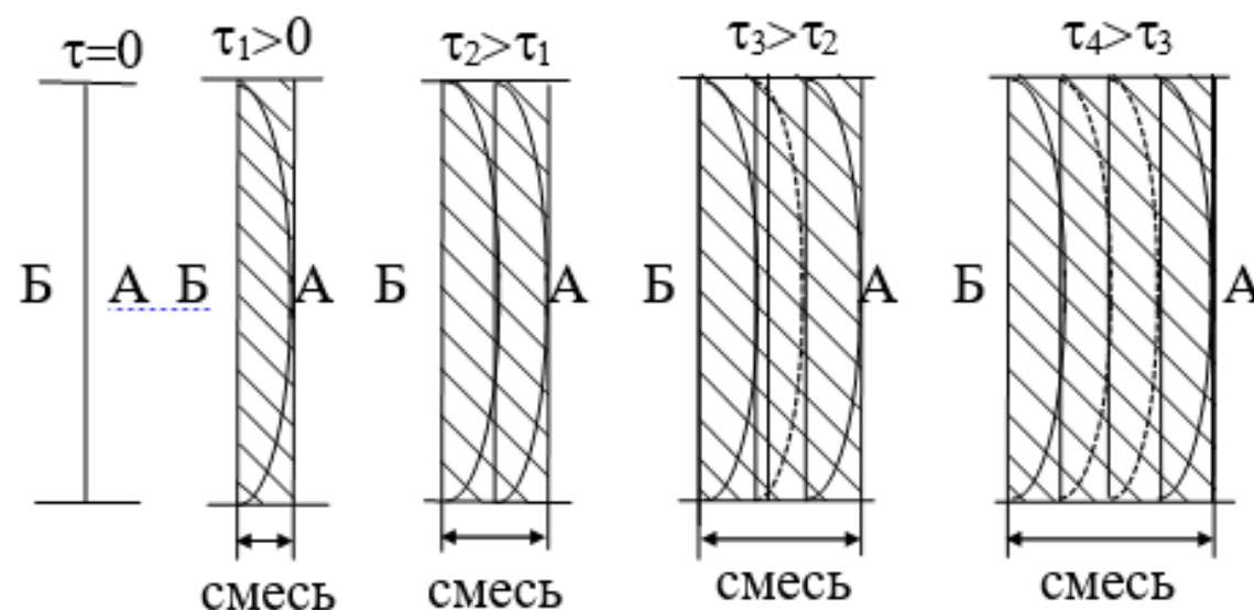
Рисунок 1.3 - Изменение объема смеси и концентрации жидкости Б по ее длине во времени
