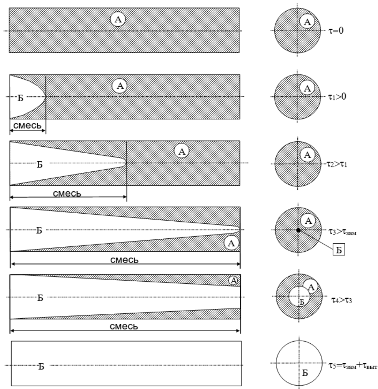
Рисунок 1.1 - Изменение объема смеси при ламинарном режиме последовательной перекачки
