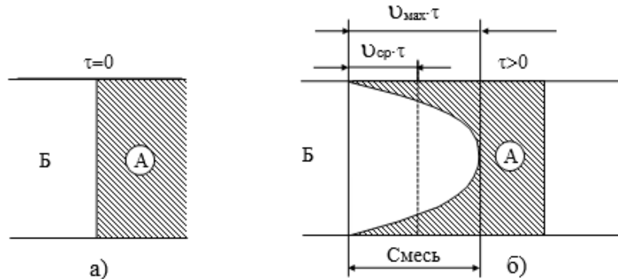
Рисунок 1 – Смесеобразование при ламинарном течении
