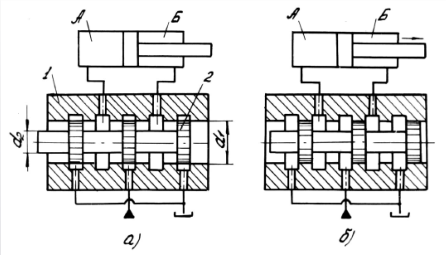
Рисунок 14.2 - Схема золотникового гидрораспределителя
