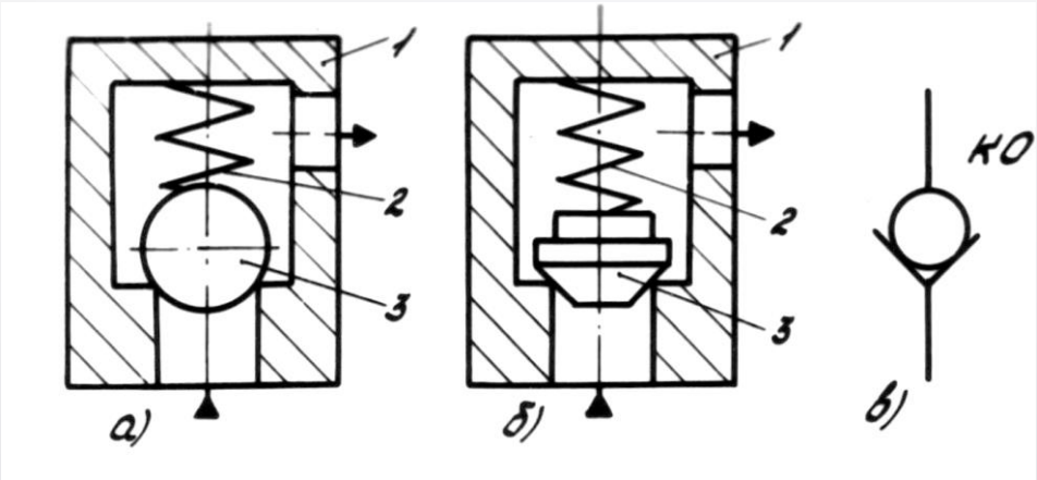
а – шарикового типа: 1 – корпус; 2 – пружина; 3 – шарик; б – конусного типа: 1 – корпус; 2 – пружина; 3 – конус; в – условное обозначение
