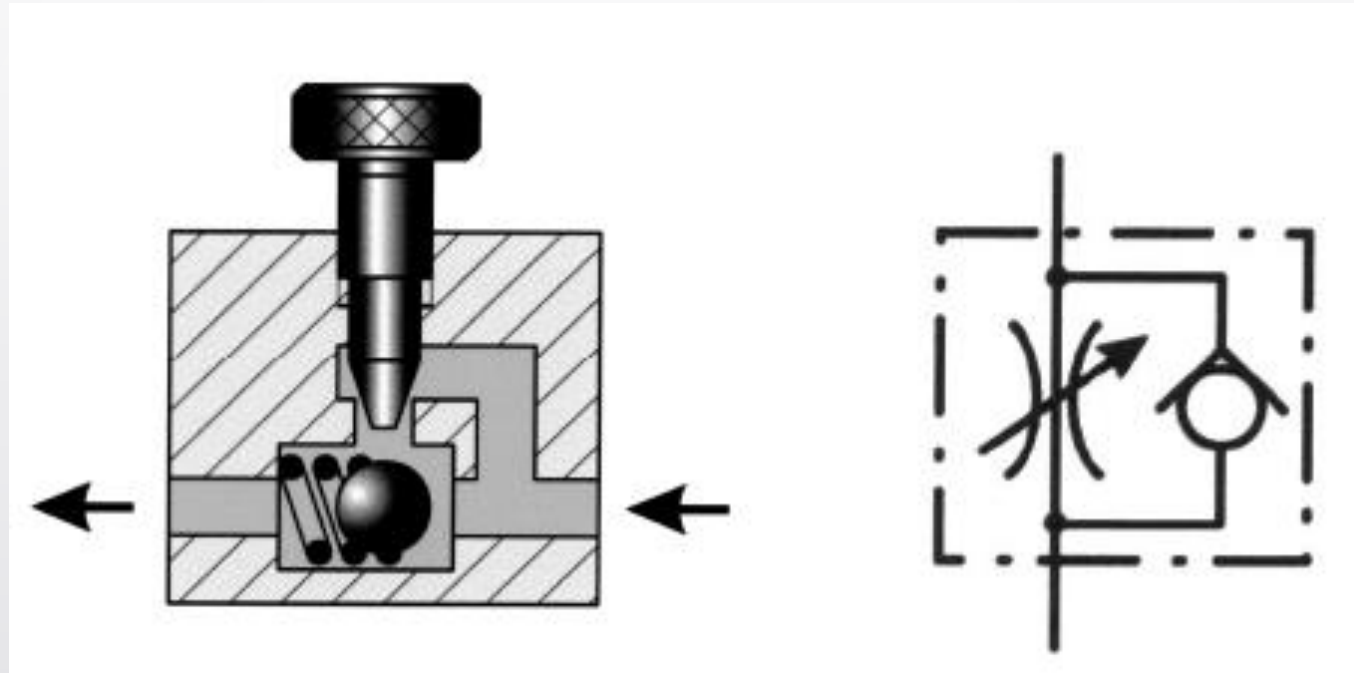
Рисунок 14.5 – Дроссель
