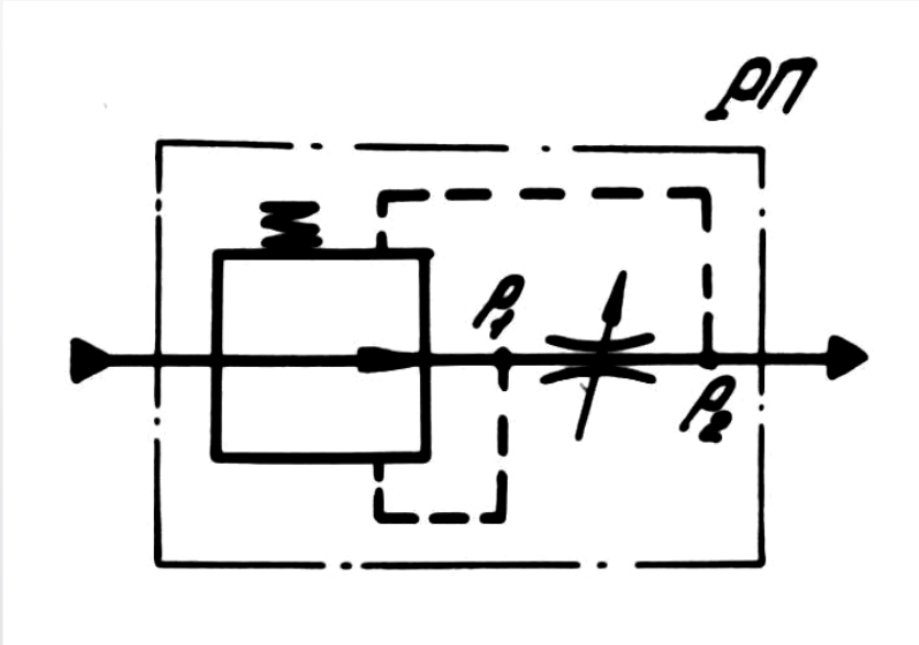
Рисунок 14.6 – Регулятор потока
