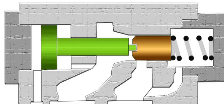
Управляемый обратный клапан Гидрозамок
