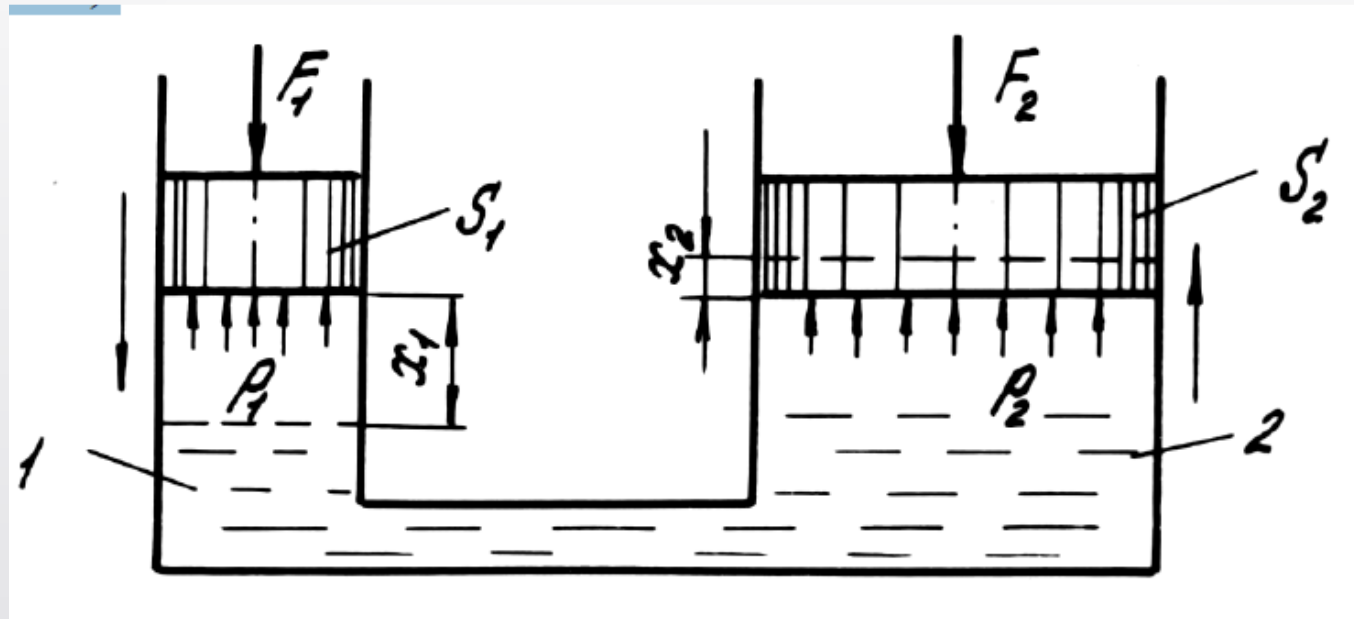
Рисунок 11.2 - Принципиальная схема простейшего объемного гидропривода
