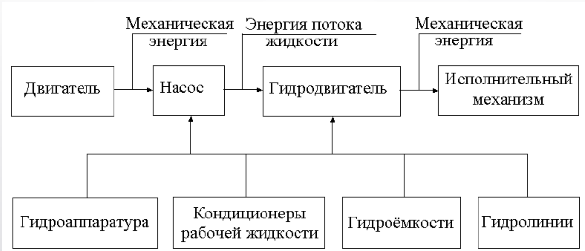
Рисунок 11.1- Функциональная схема гидравлического привода
